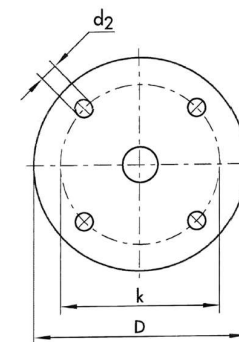
Bild: Flansch-Anschlussmaße PN 63 bis PN 320
