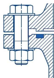
Form TG Mit Nut und Feder
