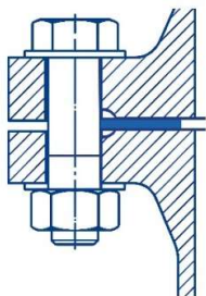
Form IBC Ebene Dichtleiste Mit und ohne Dichtleiste
