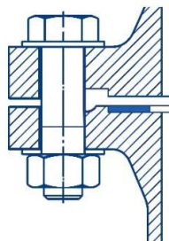
Form SR Mit Vor- und Rücksprung
