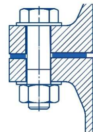
Form FF Mit Schraubenlöchern
